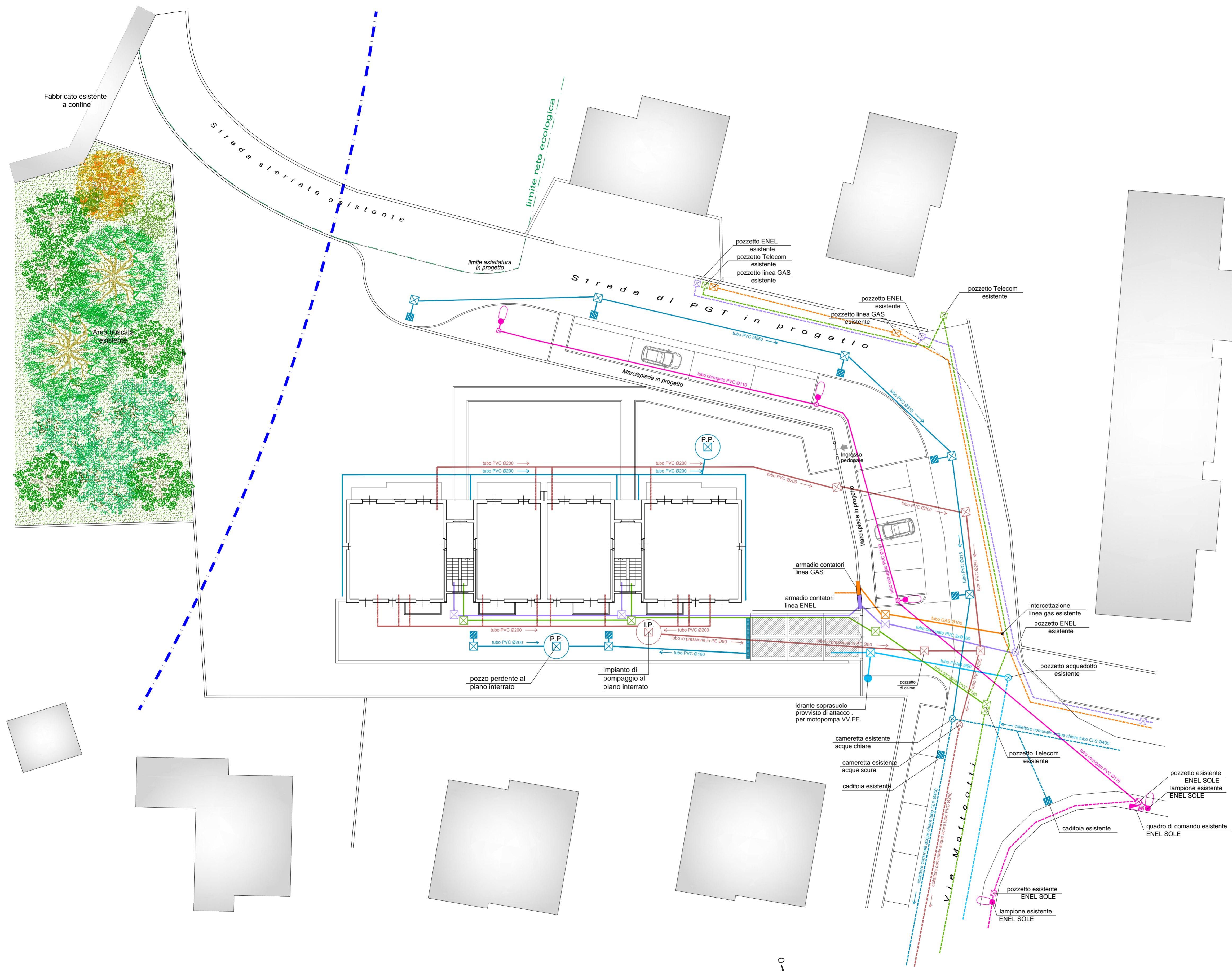
Planimetria Generale 1:200 Urbanizzazioni
